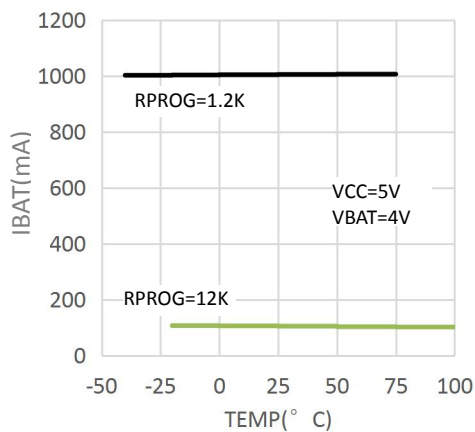
充电电流与环境温度的关系曲线
